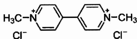
ภาพที่ 8 โครงสร้างโมเลกุลของพาราควอต
